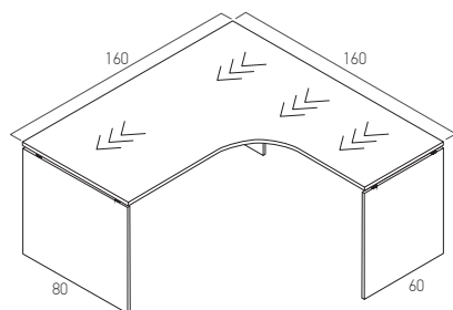
С боковиной 60/80. Правый TES 284 167 160x160xh75
