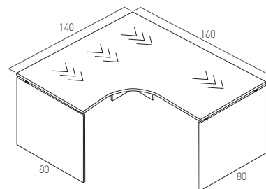
С боковиной 80. Левый TES 284 160 160x140xh75
