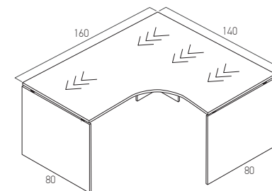
С боковиной 80. Правый TES 284 161 160x140xh75
