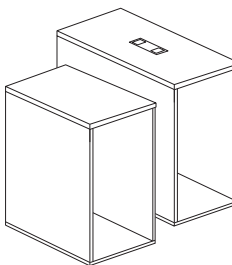
Тумба опорная под системный блок TES 284 324 35x60xh63 TES 284 325 35x80xh63
