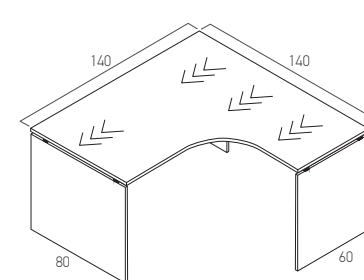
С боковиной 60/80. Правый TES 284 169 140x140xh75
