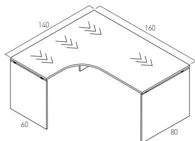
С боковиной 60/80. Левый TES 284 162 160x140xh75
