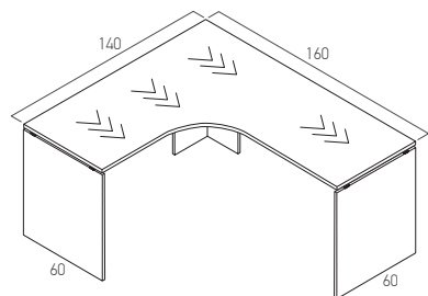
С боковиной 60. Левый TES 284 164 160x140xh75
